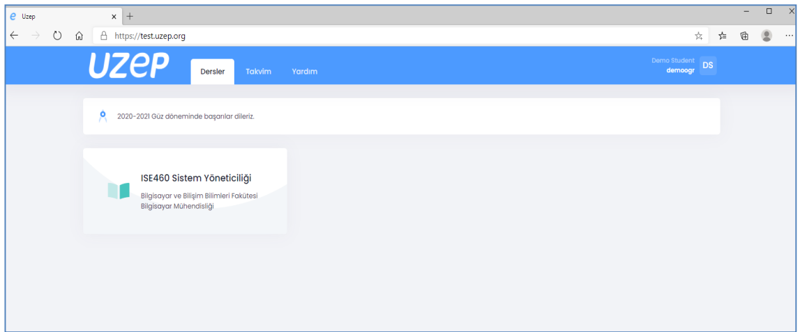
Şekil 3. Dersler Arayüzü
