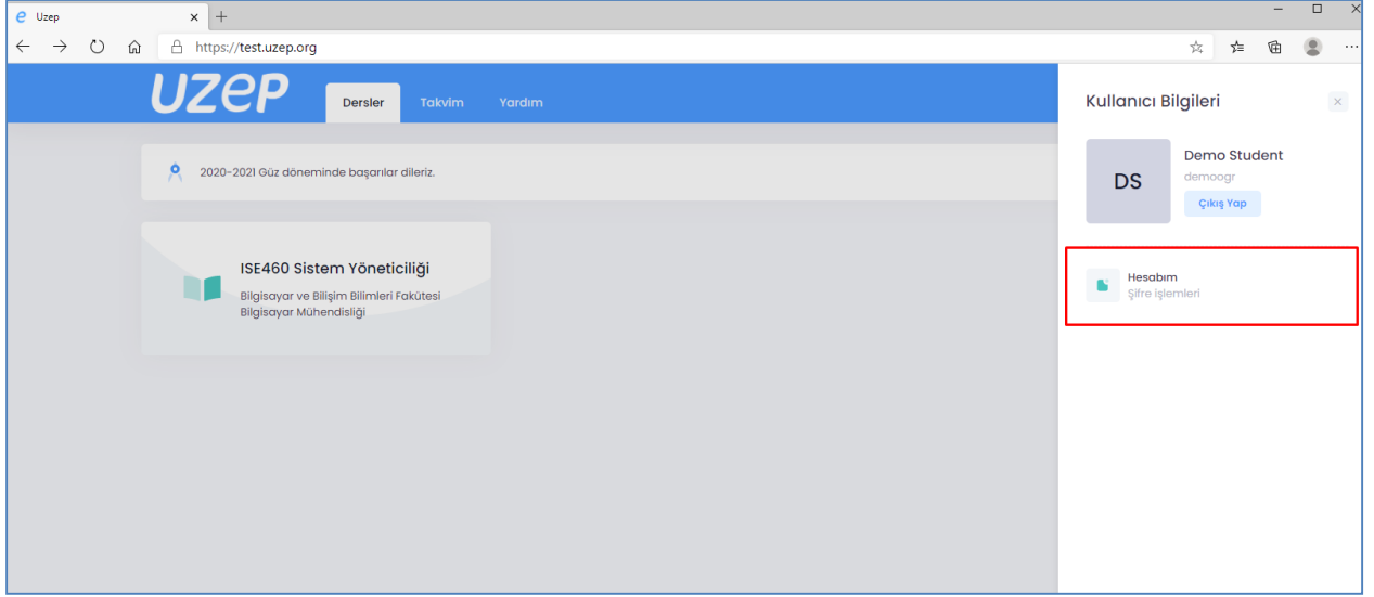
Şekil 2. Şifre güncelleme.
